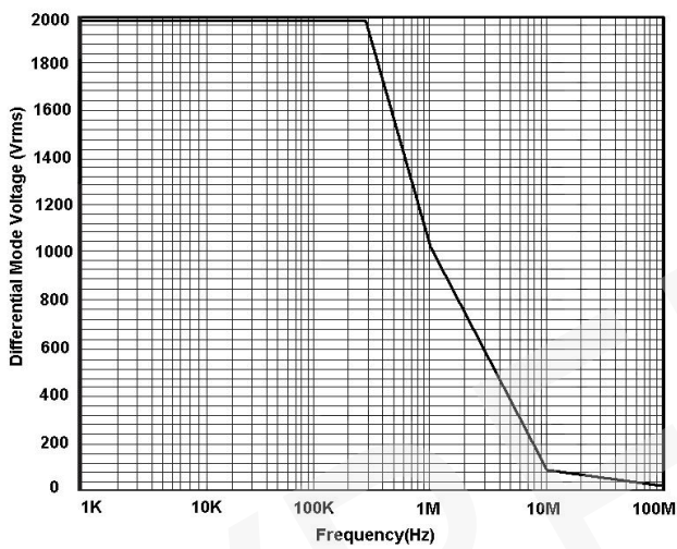
图 3: DP6350D 最大差模电压 VS 频率
